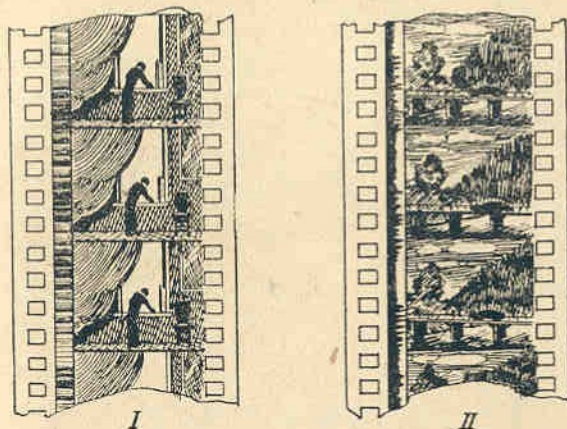
Рис. 8. Кусок киноплёнки со звуковой дорожкой: I — глубинная запись звука; II — поперечная запись.
