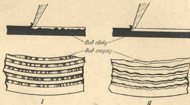
Рис. 3. Вид звуковой бороздки: I — у фонографа; II — у граммофона.
