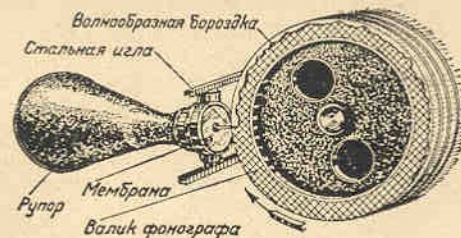
Рис. 2. Так выглядит звуковая бороздка на оловянном листе фонографа.
