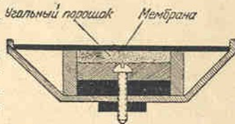
Рис. 5. Схема простейшего микрофона.
