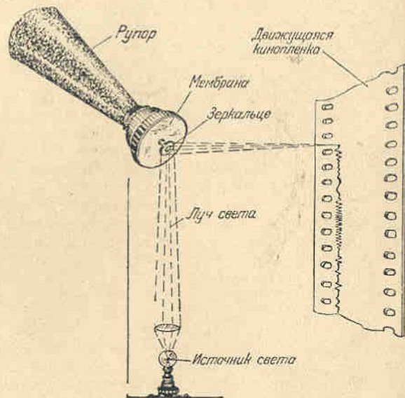
Рис. 7. Схема световой записи звука с помощью зеркала.
