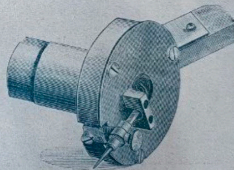
Репродукторъ съ заключенной въ немъ мембраной, изобрѣтателя граммофона проф. Э. БЕРЛИНЕРА.
