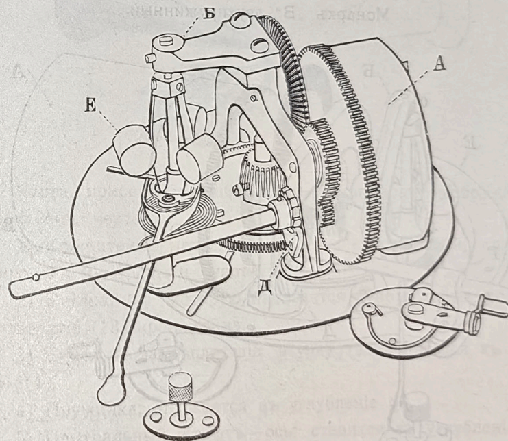
Монархъ „С“ однопружинный.
