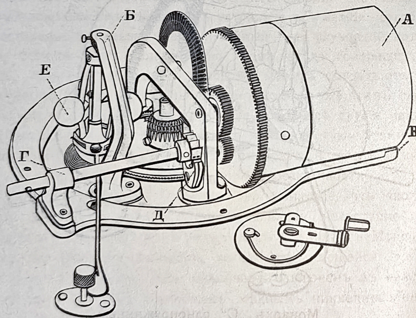
Монархъ „А“, трехпружинный.
