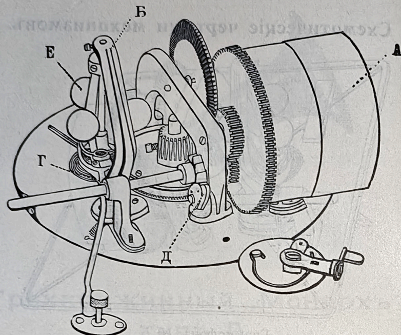
Монархъ „В“ двухпружинный.
