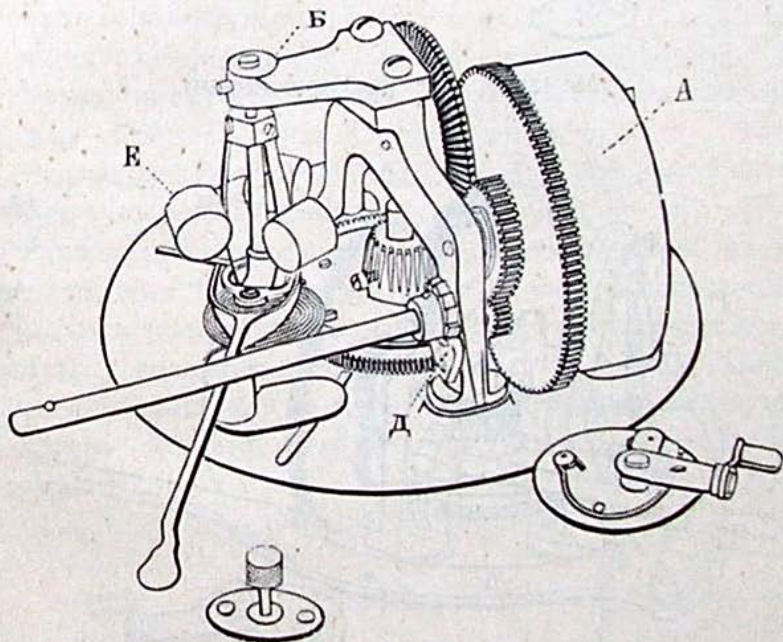
Монархъ „С“ однопружинный.
