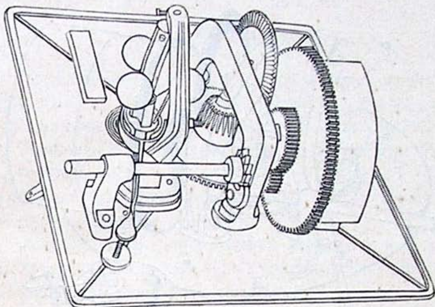
Граммофонъ № 6 „Универсаль“.
