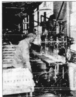
8. Сверленіе дырокъ для пробокъ въ деревянныя доски, употребляемыя при упаковкѣ аппарата для защиты таковъ отъ толчковъ.
