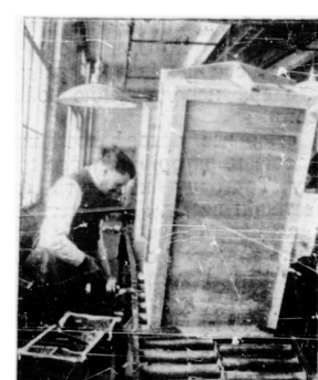
32. Сверленіе дырокъ въ упаковочн. ящикъ для прикрѣпл. нижн. досокъ, защищ. корп.
