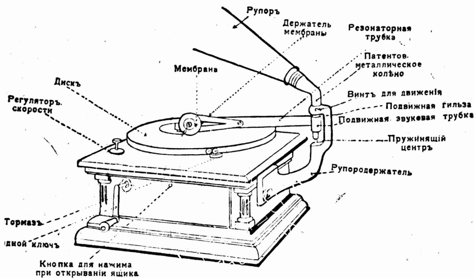
Рис. 1. Подробный чертежъ устройства «ТОНАРМА».
