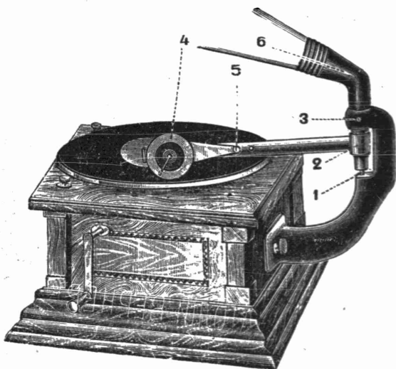
Рис. 2. Граммoфонъ «ТОНАРМЪ».
