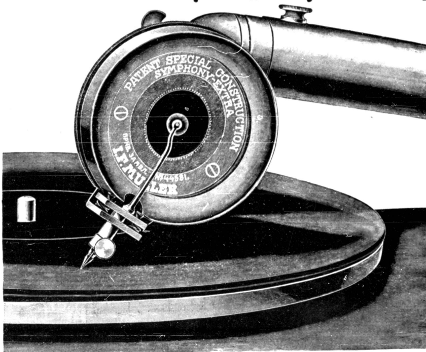
Рис. 1. Мембрана „СИМФОНИЯ-ЭКСТРА“ въ вертикальномъ положеніи съ вставленной иглой. для игры граммофонныхъ пластинокъ.
