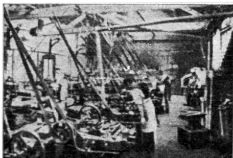
Станки въ моментъ работы по изготовленію иглъ.
