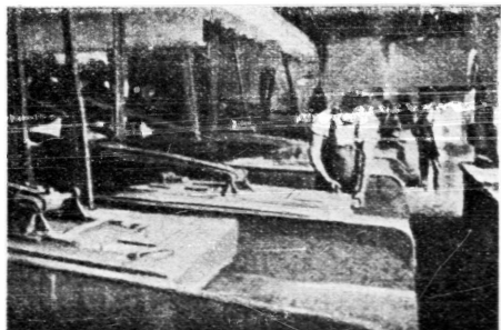
Прокатная машина, производящая полировку иглъ. Ихъ прокатываютъ четыре дня вмѣстѣ съ наждакомъ и масломъ.
